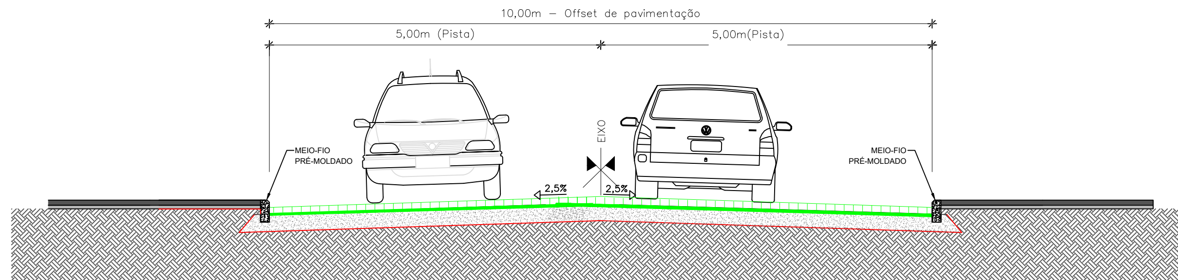
SEÇÃO TIPO DE PAVIMENTAÇÃO- Offset de pavimentação com bloco intertravado-RUA PADRE INÁCIO EIDT
